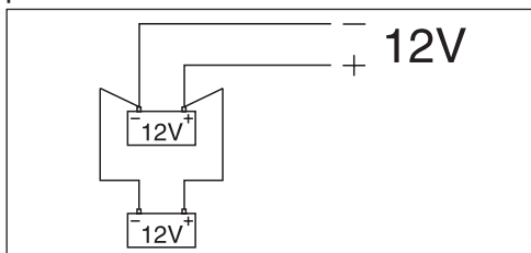
parallelforbindelse
