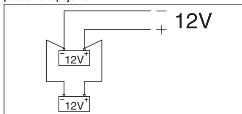
paralelné zapojenie
